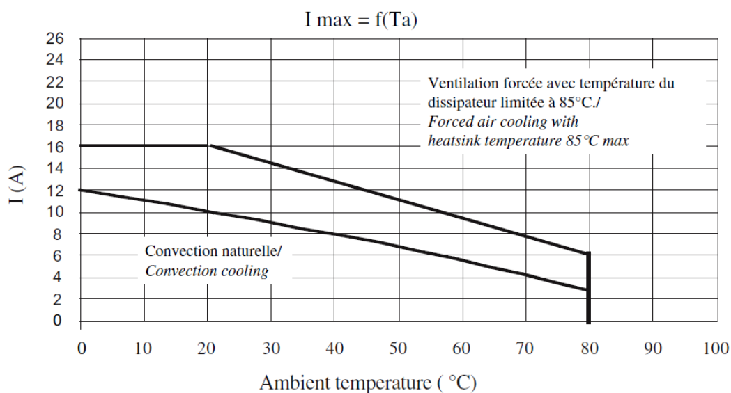
Fig.2 Caractéristiques thermiques / thermal curves :
