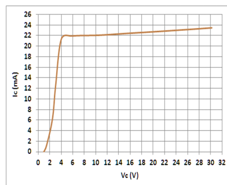
Fig.1 : Input Ic = f (Uc)
